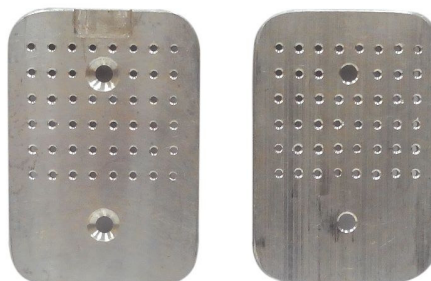
Вакуумная планка
